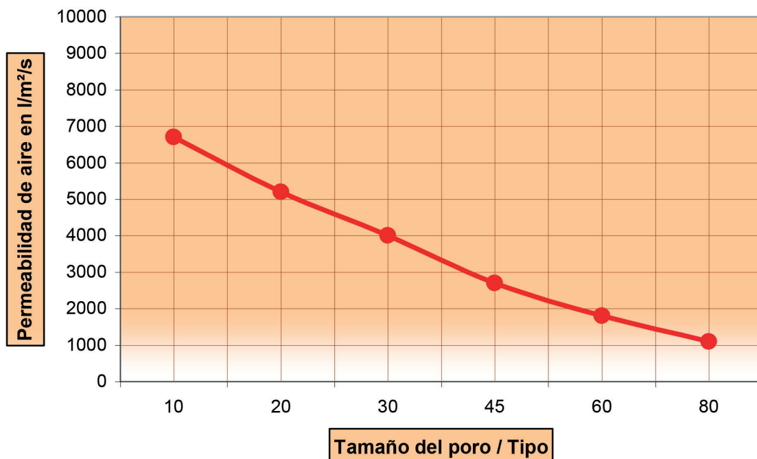
PERMEABILIDAD AL AIRE DEL ESCOESP PPI 30 PARA UNA PÉRDIDA DE CARGA DE 100Pa
